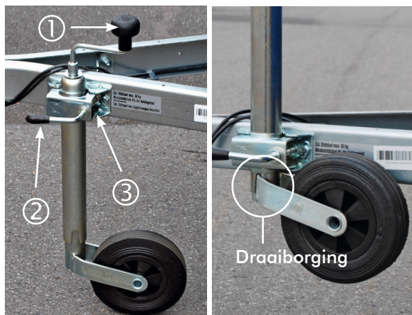
Foto rechts: Correct omhoog geplaatst steunwiel
