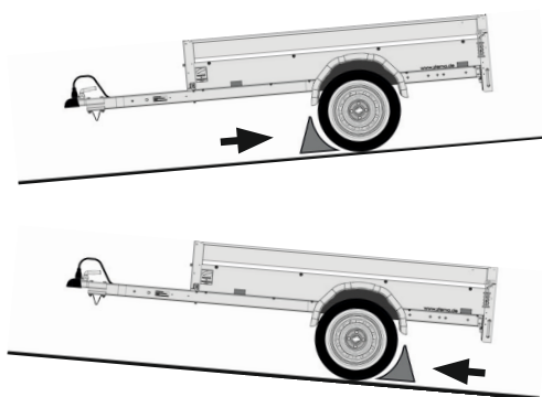
Onderlegblokken om in hangpositie te borgen
