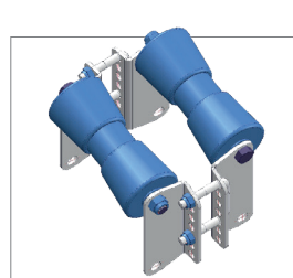
Tandem-Kielrollen mit Halterung
