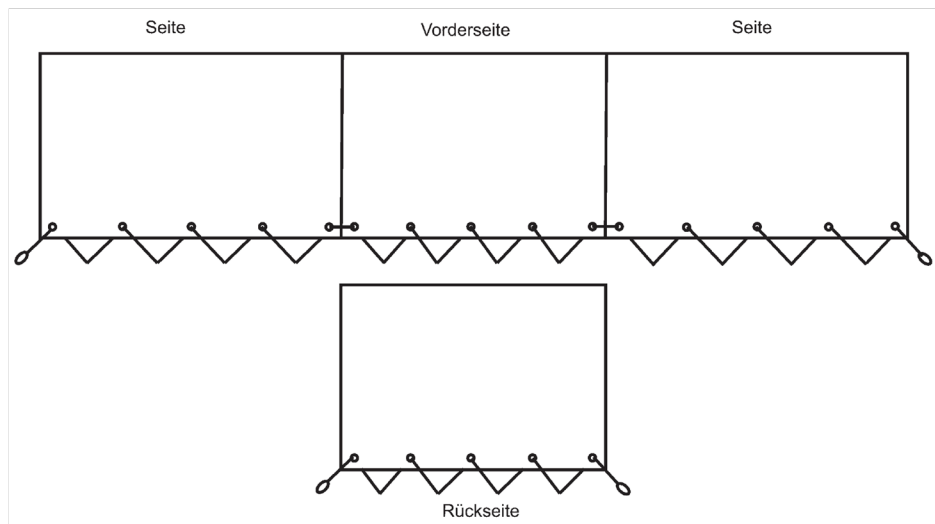
Befestigung der Planenschnur für die Rückseite der Hochplane
