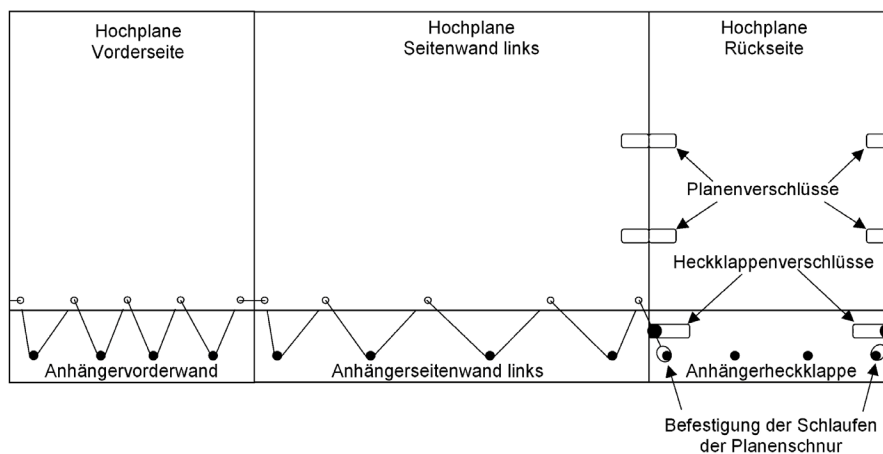
Befestigung der Planenschnur für die Rückseite der Hochplane
